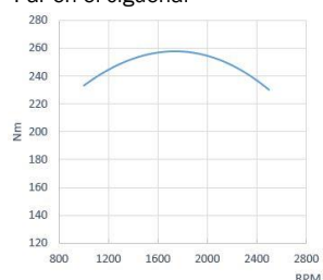
Par en el cigüeñal
